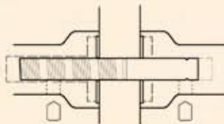
Fissaggio UG per paio maniglioni Back-to-back fixing
